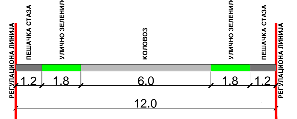
ПОПРЕЧНИ ПРОФИЛ ПРИСТУПНЕ САОБРАЋАЈНИЦЕ IV-IV P=1:100
